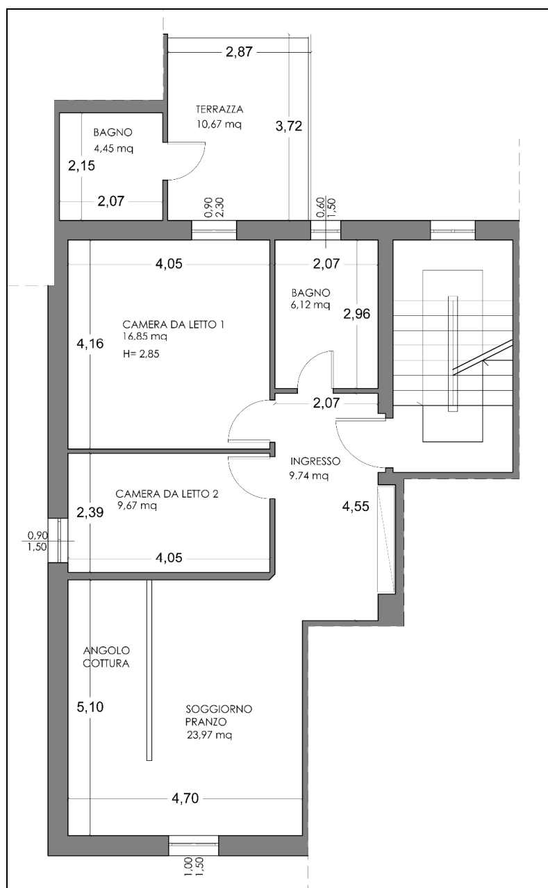
Figura 4 Rilievo dell'appartamento
